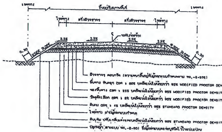
รูปตัดแสดงโครงสร้างถนนคอนกรีตเสริมเหล็กและคูระบายน้ำไว้ด้วย
