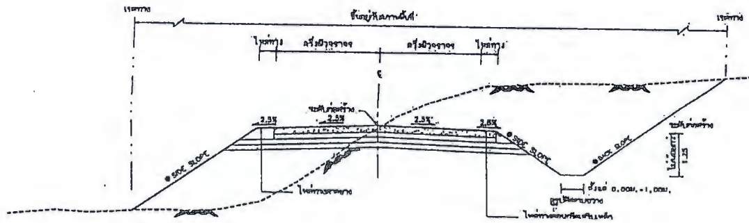
รูปตัดตามขวางแสดงดินชั้นและดินถม
